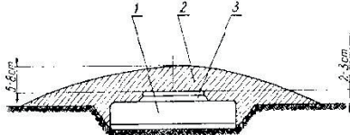
Rys. 3. Sposób ustawienia miny ppanc. w gruncie twardym: 1 – mina, 2 – warstwa maskująca minę, 3 – pokrywa naciskowa miny. Źródło: „Poradnik szeregowego zawodowego oraz szeregowego Narodowych Sił Rezerwowych” - sygn. DWLąd. Wewn. 191/2011.
