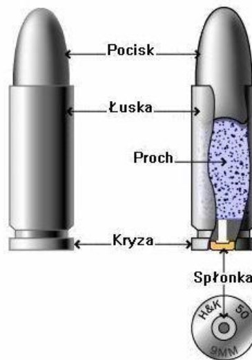
Rys. 9. Budowa naboju
