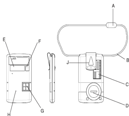
Fot. 23. Dawkomierz indywidualny SOR/T/widok płyty czołowej
