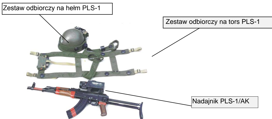
Fot. 28. Laserowy Symulator Strzelania PLS-1/AK.
