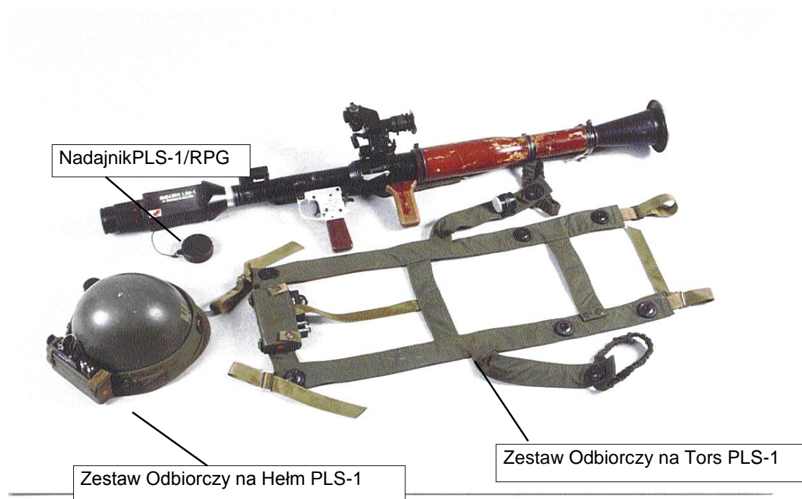
Fot. 33. Laserowy Symulator Strzelania PLS-1/RPG.
